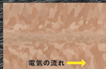
鍛造未処理の導体断面
